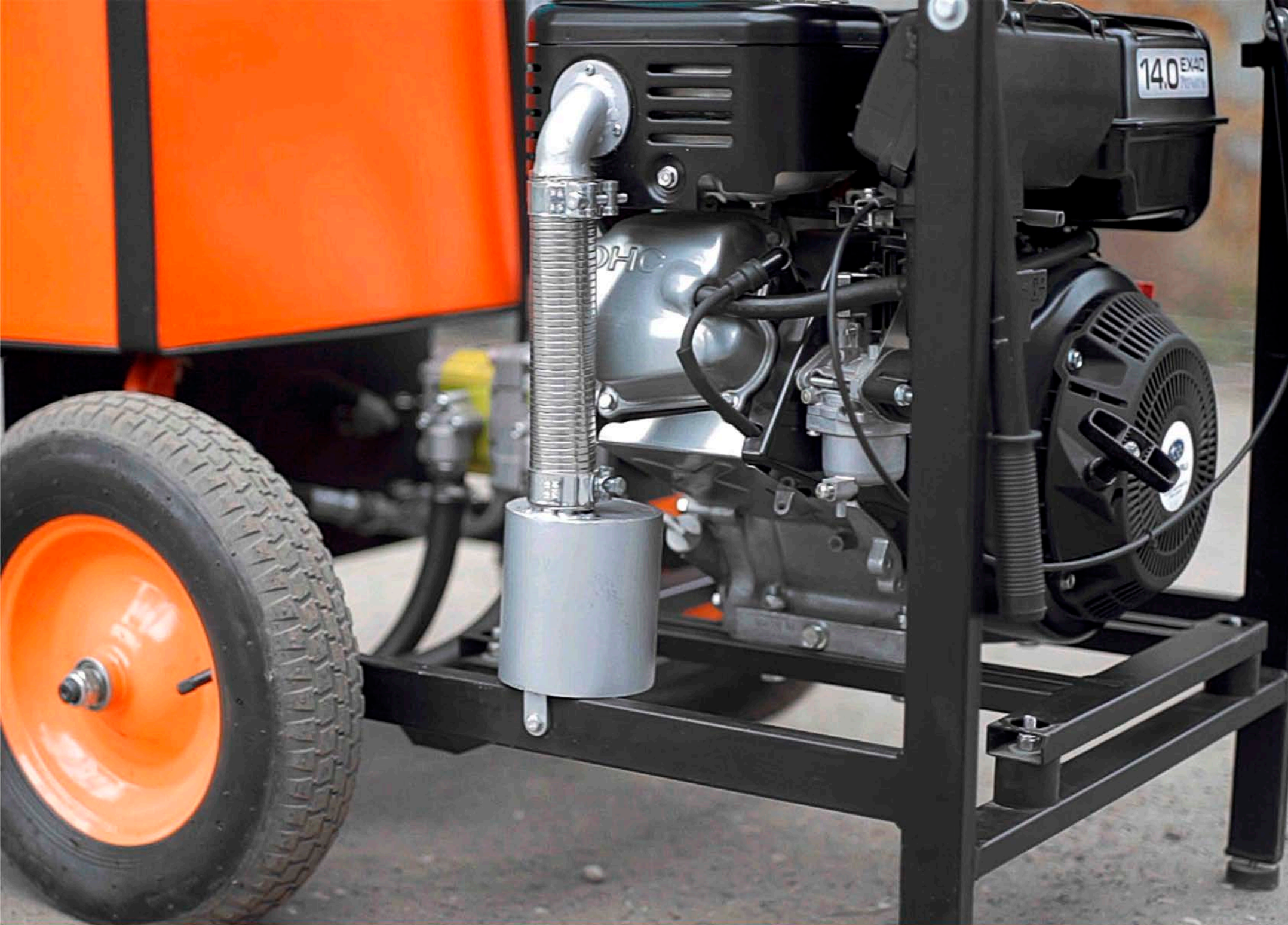
ИСКРОГАСИТЕЛЬ «ИПГ»
